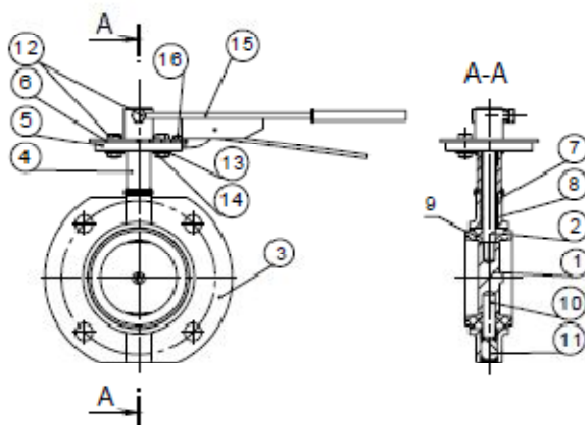
Рисунок 6.1. Затворы 32с60р: устройство и материалы
